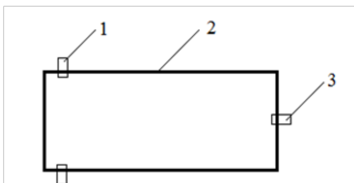
1- 称重传感器；2- 秤架；3- 称重传感器
