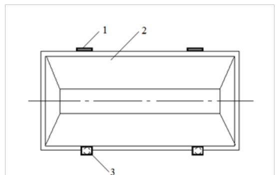
1- 铰链支撑；2- 称重料仓；3- 称重传感器
